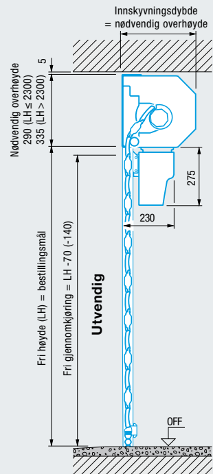
Montering i åpningen
