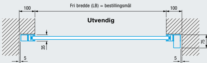
Montering bak åpningen
