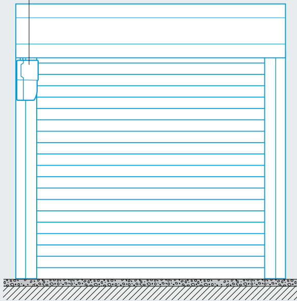
Portåpner (håndkjedetrek), innvendig venstre side
