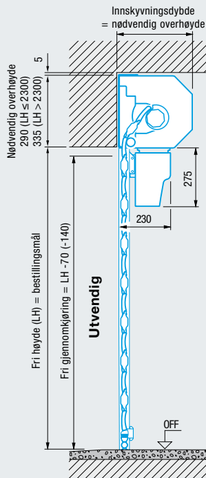
Montering bak åpningen
