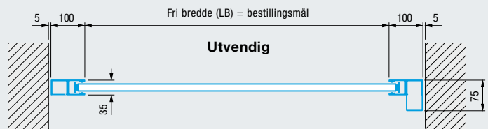
Montering i åpningen
